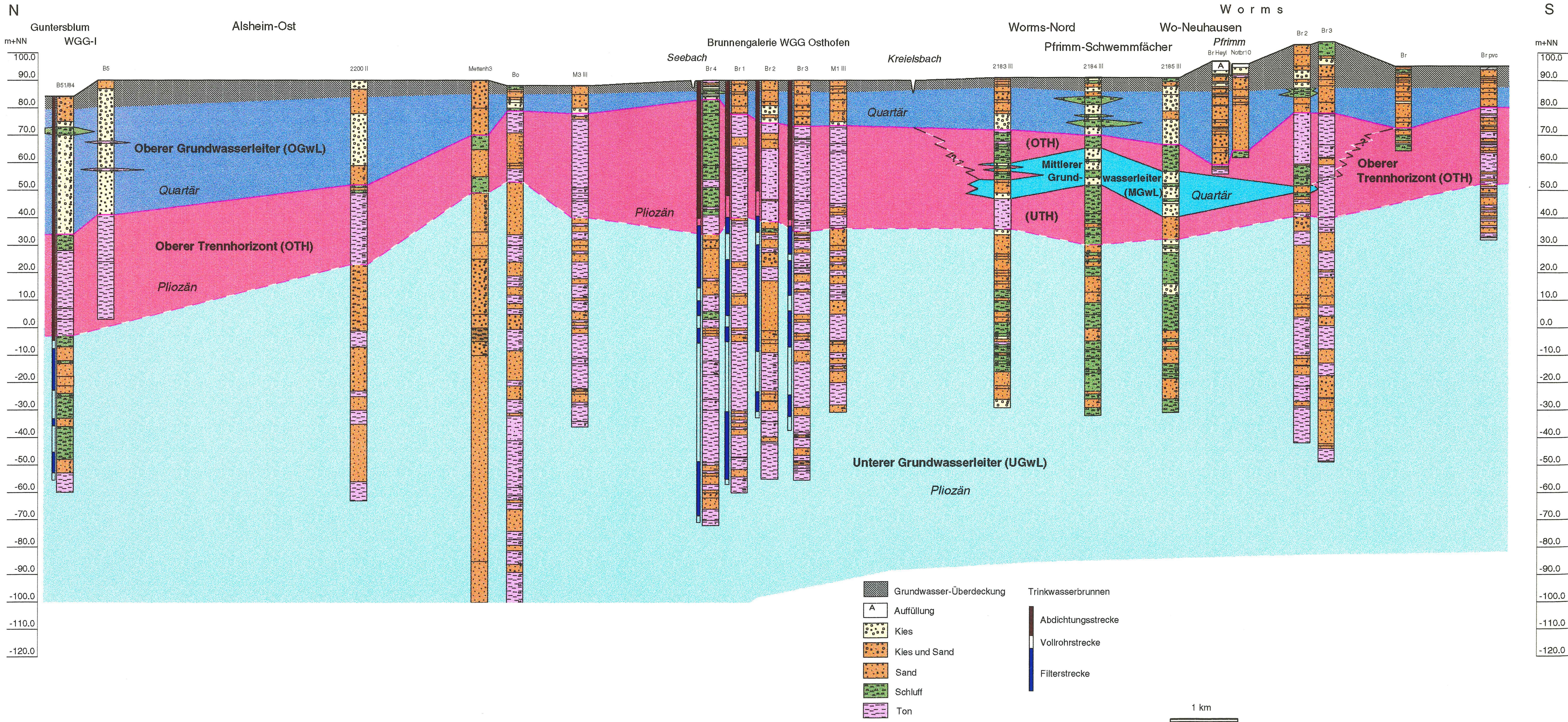
Hydrogeologischer Übersichtsschnitt L1
